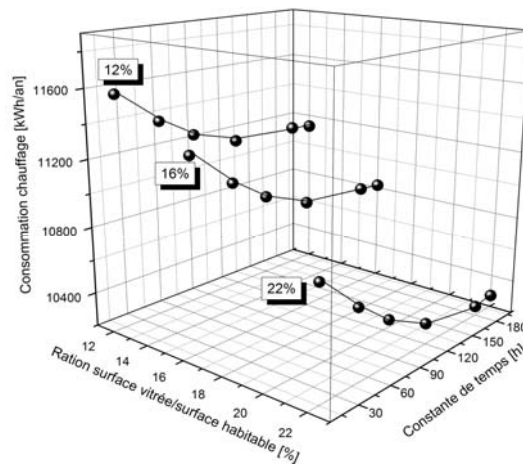
Figure 2. Impact de la morphologie et de la surface vitrée d'un bâtiment sur la consommation d'énergie pour le chauffage
